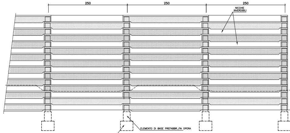
PARTICOLARE PROSPETTO
