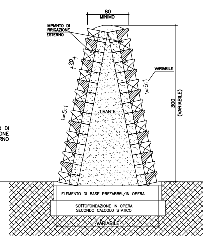
SEZIONE TIPO
