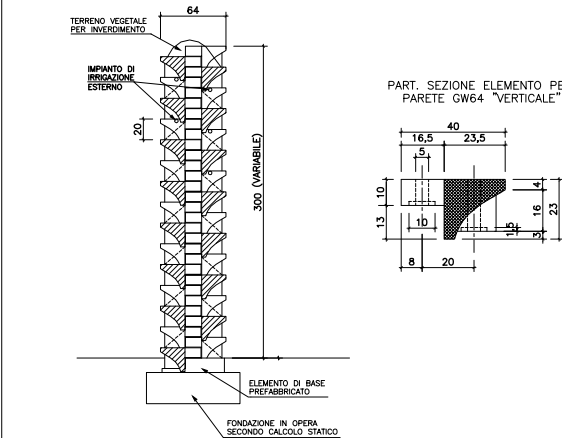
SEZIONE TIPO
